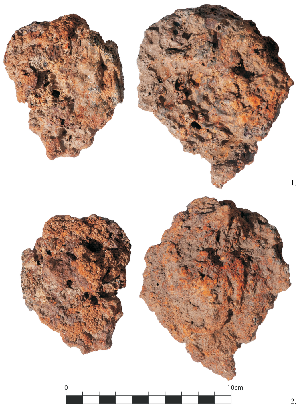
Fig. 13: Zguri de forjă descoperite în complexul 139 (152 gr. cea din stânga) și complexul 001 (428 gr. cea din dreapta). Fotografii ce arată partea de sus (1) și de jos (2) a zgurilor.
