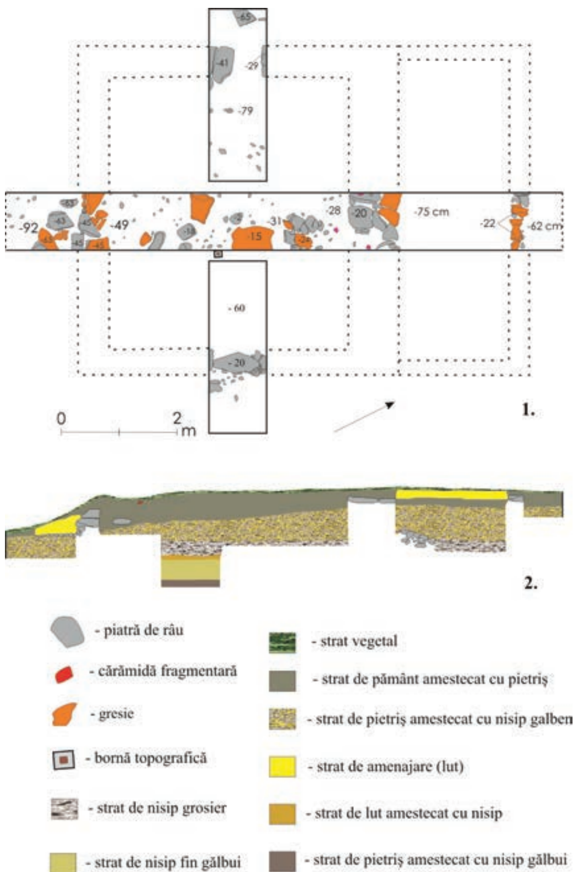
Fig. 14: Dealul Arțariș (cota 803) - planul (1) și profilul (2) fundației din piatră.
