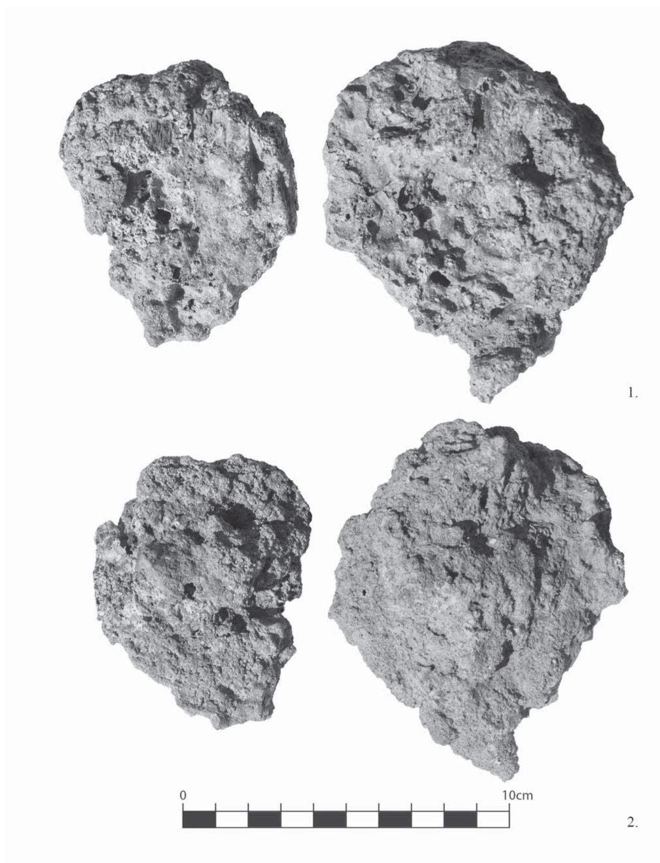
Fig. 15: Zguri de forjă descoperite în complexul 139, 152 gr. cea din stânga și 428 gr. cea din dreapta. Fotografii ce arată partea de sus (1) și de jos (2) a zgurilor.
