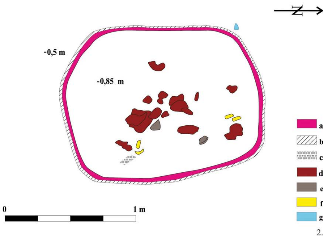
Fig. 5: Fotografie din timpul cercetării complexului 139 (1) și desen (2). Legenda: a- perete lutuit și ars; b- pământ ars (în exteriorul gropii); c- lemn carbonizat; d- material metalurgic; e-fragmente ceramice; f- oase arse; g- silex.
